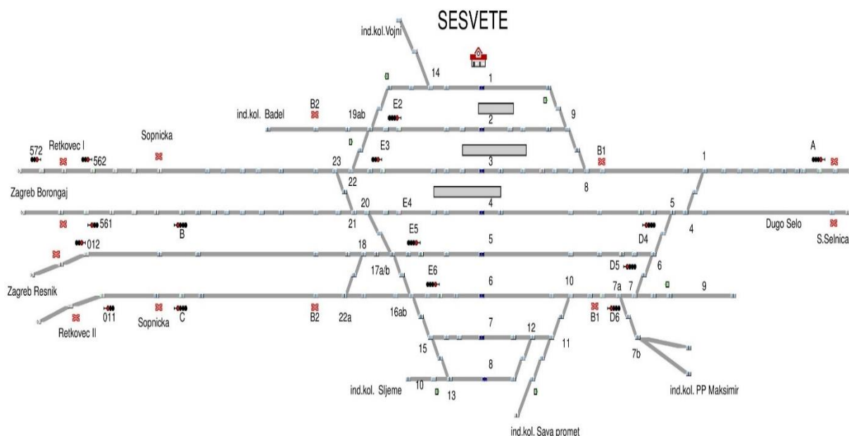
Slika 31. Prikaz kolodvora Sesvete u programskom paketu Open Track
