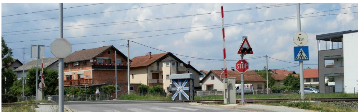
Slika 20. ŽCP „Sesvetska Selnica“
