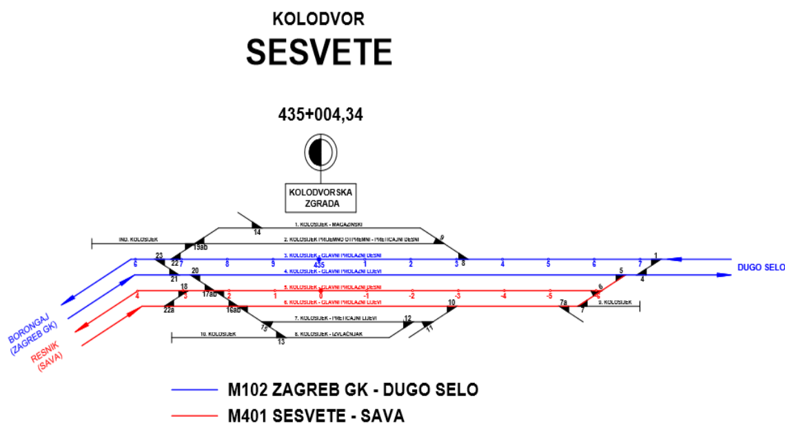
Slika 12. Shema kolodvora Sesvete, [2]
