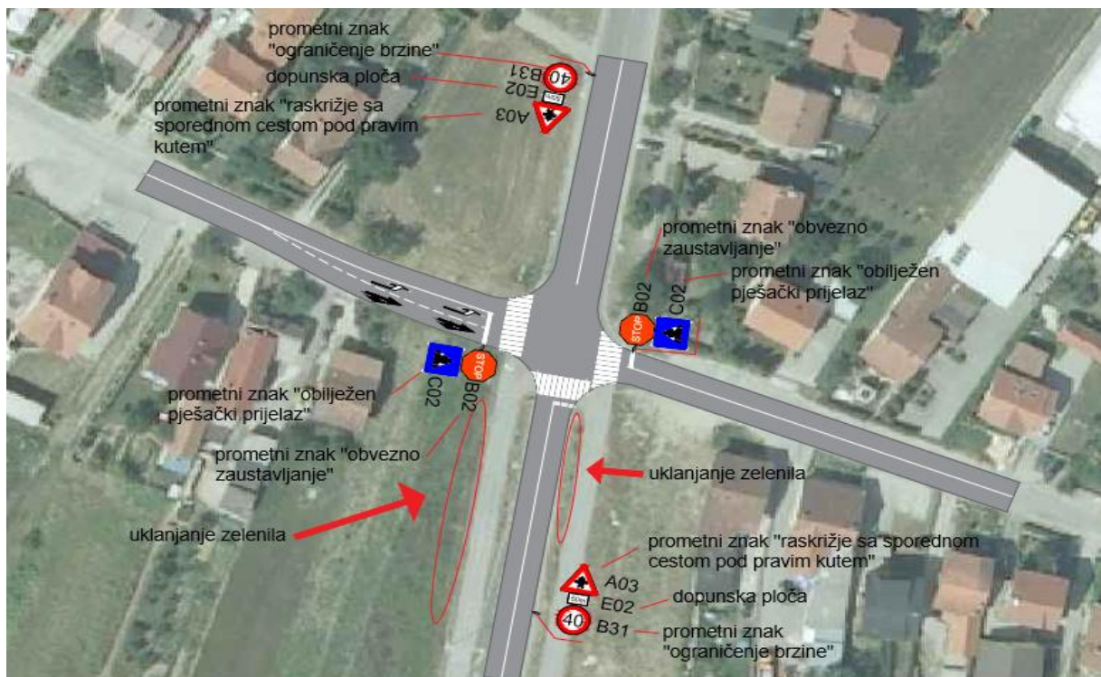
Slika 75. Idejno rješenje za raskrižje ulica Slavka Kolara i Nikole Tesle - Varijanta 1
