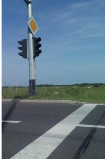
Slika 64. Puna crta zaustavljanja
